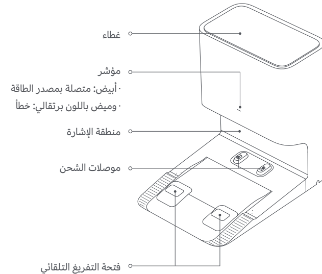
العرض الأمامي
