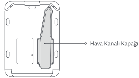
Alttan Görünüm
