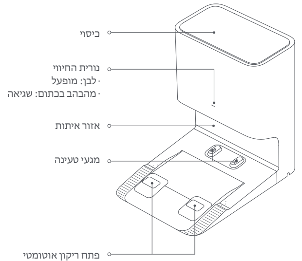
מבט מלפנים
